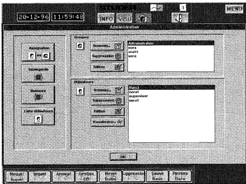
Abb. 4: «Zugangsrechte-Module»
